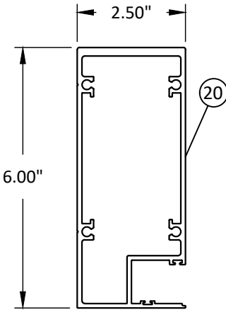
JAMB - 'J1'
