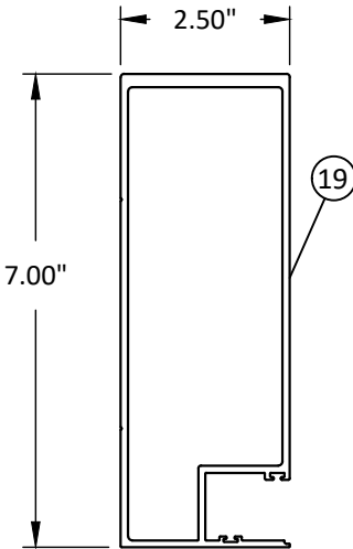
JAMB - 'J3'
