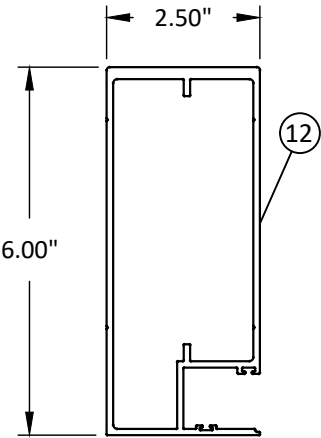
JAMB - 'J2'
