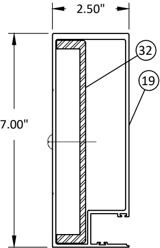
JAMB - 'J4'
